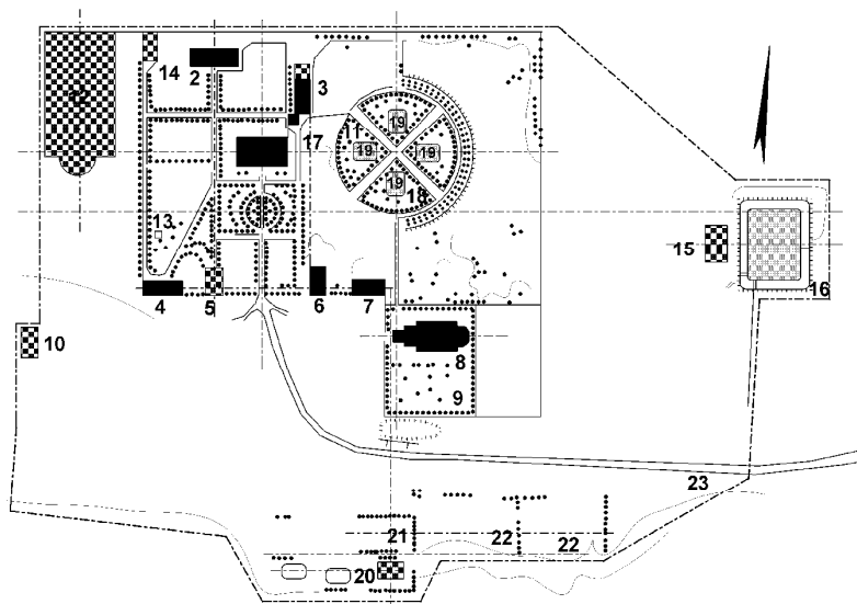
Рис. 4. Усадьба Нероново (Россия). Генплан: 1 – главный дом; 2 – дом управляющего; 3 – хозяйственный флигель; 4 – дом помощника управляющего; 5 – амбар; 6 – баня; 7 – сторожка; 8 – церковь Воскресения; 9 – некрополь; 10 – дом священника; 11 – место паркового павильона; 12 – скотный двор; 13 – колодец; 14 – каретный сарай; 15 – прачечная; 16 – большой пруд; 17 – плодовый сад; 18 – «водный партер»; 19 – пруды; 20 – место грунтового сарая; 21 – место оранжереи и ягодного сада; 22 – хозяйственный двор; 23 – подъездная дорога
