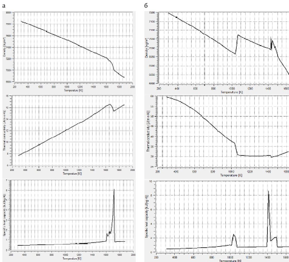
Рис. 6. Расчетные зависимости плотности (density), теплопроводности (thermal conductivity) и теплоемкости (specific heat capacity) в зависимости от температуры для 08X19H10T (а) и ВЧШГ (б)
