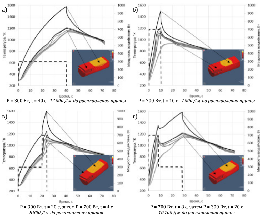
Рис. 11. Температуры в зонах непосредственного ЭЛ воздействия (верхние графики) и зонах пайки (нижние графики) при различных циклограммах (пунктирная линия) теплового воздействия ( P – мощность, t – продолжительность)
