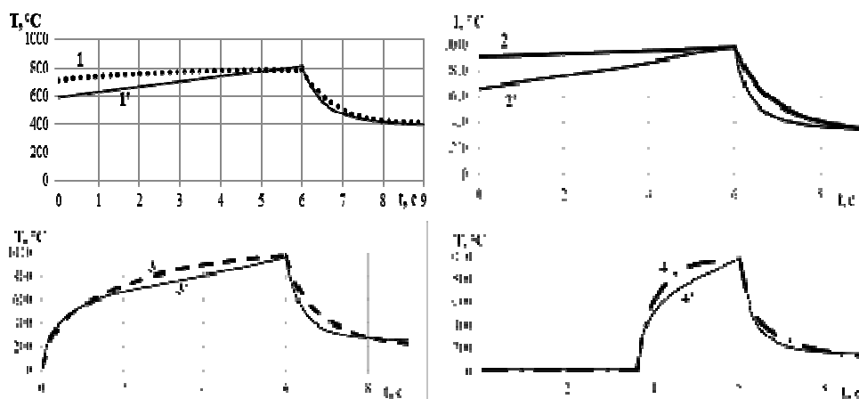
Рис. 3. Совмещенные графики температур экспериментальных образцов и результатов КЭ моделирования
