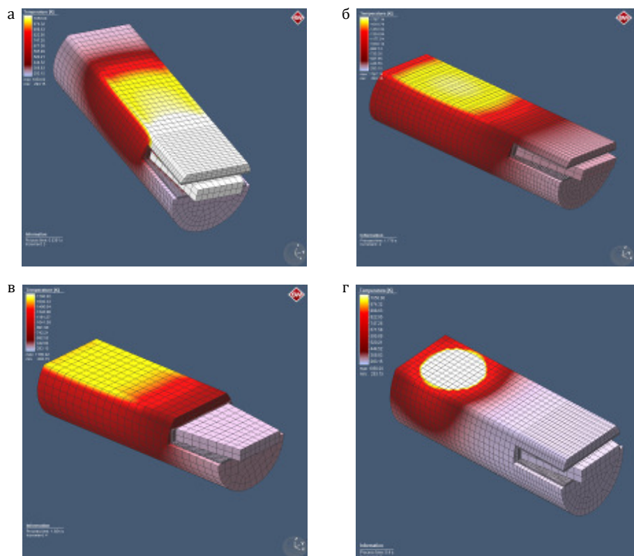
Рис. 10. Распределение тепловых полей в модели электронно-лучевой пайки оправки режущего инструмента при различных размерах и областях воздействия источника тепла: а) воздействие на участок, близлежащий к паяемому соединению; б) воздействие на заднюю часть оправки; в) модель оправки без открытого паза; г) воздействие пучком диаметром 5 мм
