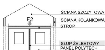
Rys. 6. Schemat zamontowanego słupa żelbetowego (etap 2)
