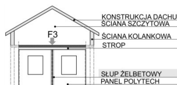
Rys. 7. Schemat zamontowanego słupa żelbetowego (etap 3)
