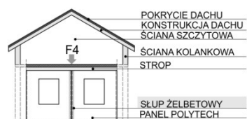
Rys. 8. Schemat zamontowanego słupa żelbetowego (etap 4)
