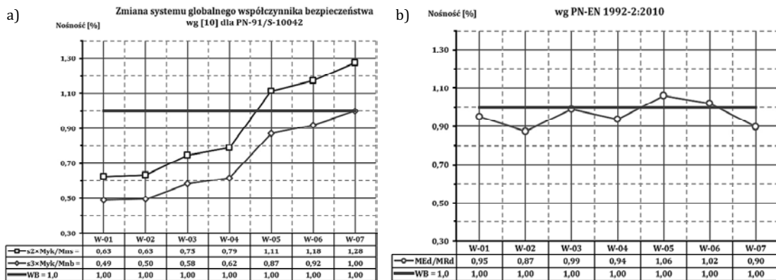
Rys. 5. Wykresy nośności przęsła mostowego: a) wg normy PN-91/S-10042 przy zmianie systemu globalnego współczynnika bezpieczeństwa dla warunku (1), gdzie s_2 = 1,52 wg [10], oraz dla warunku (2), gdzie s_3 = 1,80 wg [10]; b) wg normy PN-EN 1992-2:2010 [6] zgodnie z warunkiem (4), bez współczynników bezpieczeństwa w normie [5]
