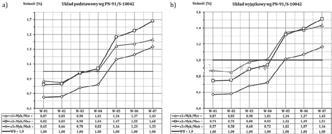
Rys. 4. Wykresy nośności przęsła mostowego wg normy PN-91/S-10042 przy zastosowaniu obliczeń: a) dla układu podstawowego, gdzie współczynniki bezpieczeństwa wynoszą odpowiednio: s_1 = 1,2 , s_2 = 2,0 i s_3 = 2,4 ; b) dla układu wyjątkowego, gdzie współczynniki bezpieczeństwa wynoszą odpowiednio: s_1 = 1,2 , s_2 = 1,8 i s_3 = 2,1
