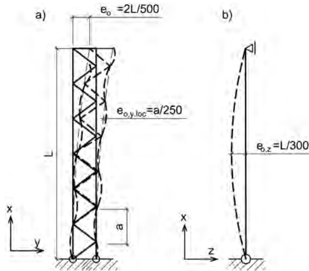
Rys. 5. Wstępne imperfekcje słupa dwugłęziowego wg [1]: a) w płaszczyźnie zginania xz, b) w płaszczyźnie xy
