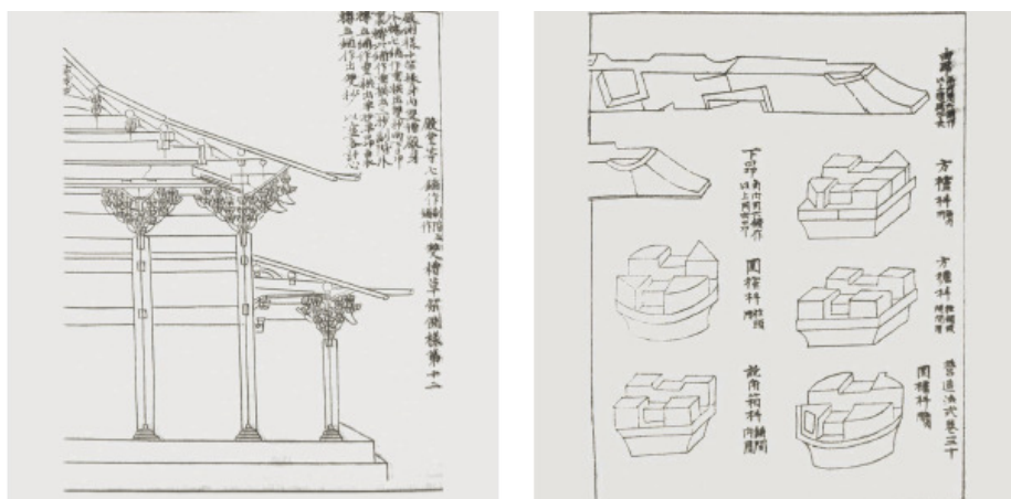
Рис. 3. Каркас и консоли жилого дома по као-гун-цзи
