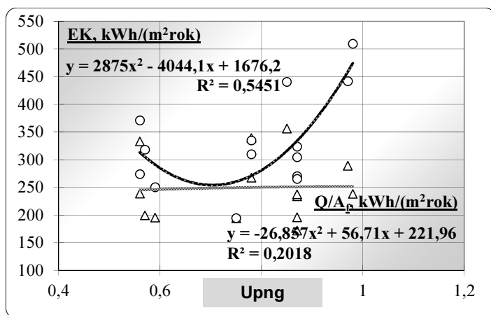
Rys. 3. Wpływ współczynnika przenikania podłogi na gruncie na EK i Q/A p
