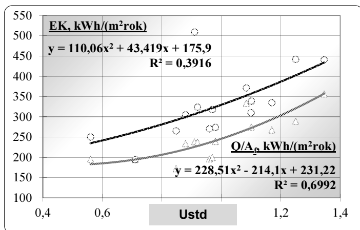
Rys. 2. Wpływ współczynnika przenikania ciepła stropodachu na EK i Q/A p
