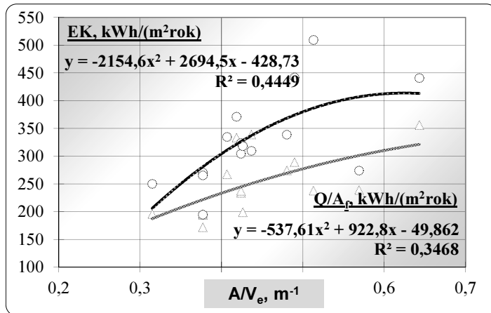
Rys. 5. Wpływ współczynnika zwartości na EK i Q/A_f
