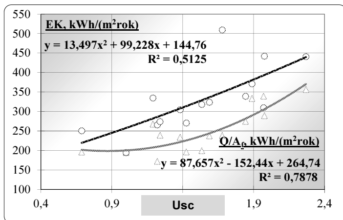
Rys. 1. Wpływ współczynnika przenikania ciepła ściany na EK i Q/A p
