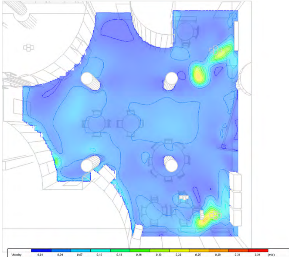
Rys. 4. Rozkład prędkości strug powietrza w pomieszczeniu A na wysokości 1,1 m
