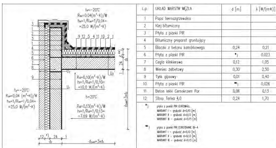
Rys. 2. Charakterystyka materiałowa połączenia stropodachu pełnego ze ścianą zewnętrzną trójwarstwową [9]
