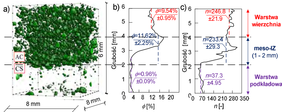
Rys. 4. Porowatość betonu w strefie zespolenia warstwy wierzchniej z podkładową określoną metodą rentgenowskiej mikrotomografii komputerowej w skali mezo:
