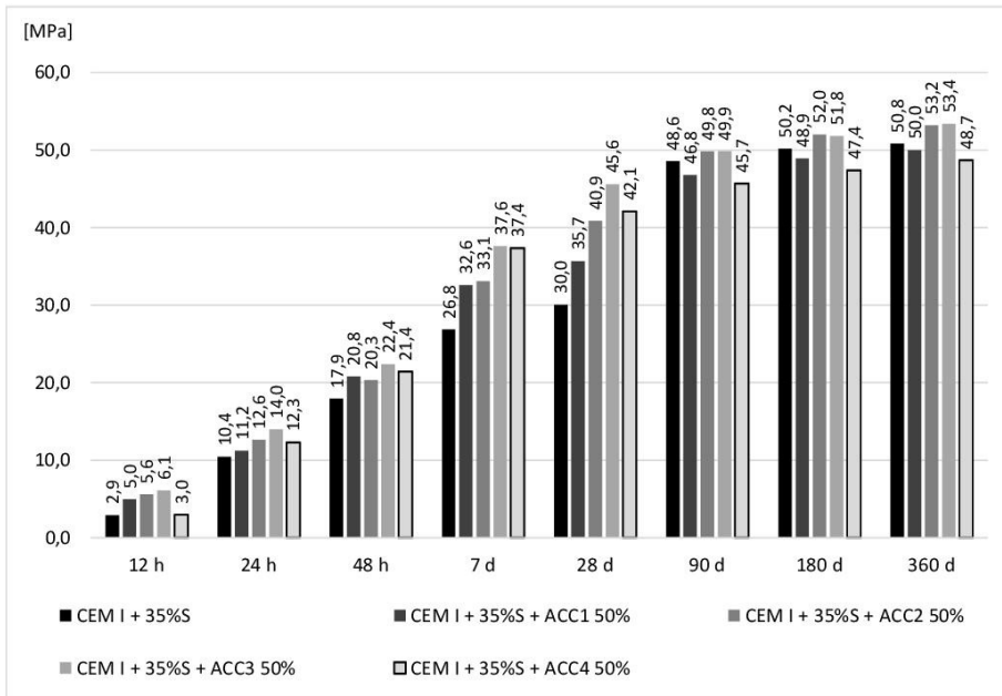
Rys. 5. Wytrzymałość na ściskanie zapraw z cemu portlandzkiego z dodatkiem 35% MGŻW w obecności połowy maksymalnej dawki domieszek
