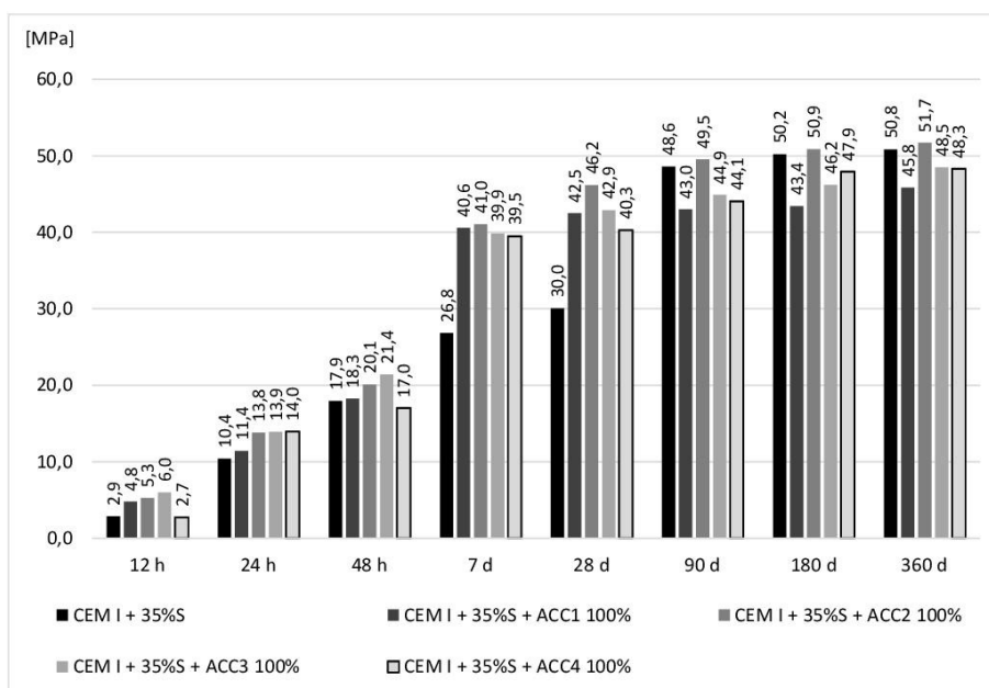
Rys. 4. Wytrzymałość na ściskanie zapraw z cementu portlandzkiego z dodatkiem 35% MGŻW w obecności maksymalnej dawki domieszek
